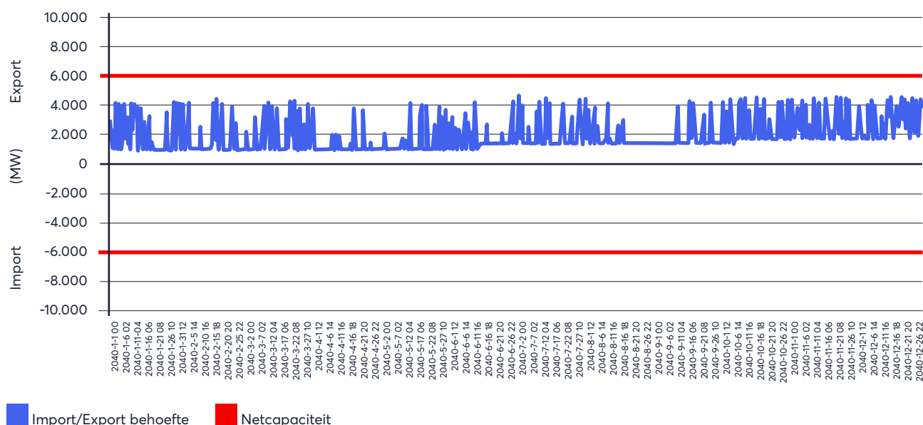
Figuur 45: Knelpuntenanalyse urniveau exportcapaciteit (1b + SV, basisjaar 2040)
