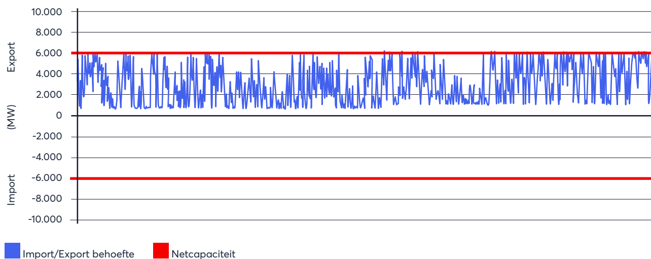
Figuur 42: Knelpuntenanalyse uurniveau exportcapaciteit (4b + SF, basisjaar 2040)
