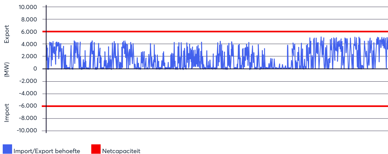
Figuur 40: Knelpuntenanalyse uurniveau exportcapaciteit (4a + SF, basisjaar 2040)
