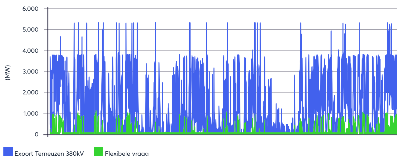
Figuur 49: Locatiesturing vraagstimulering Liechtensteinweg – Rilland
