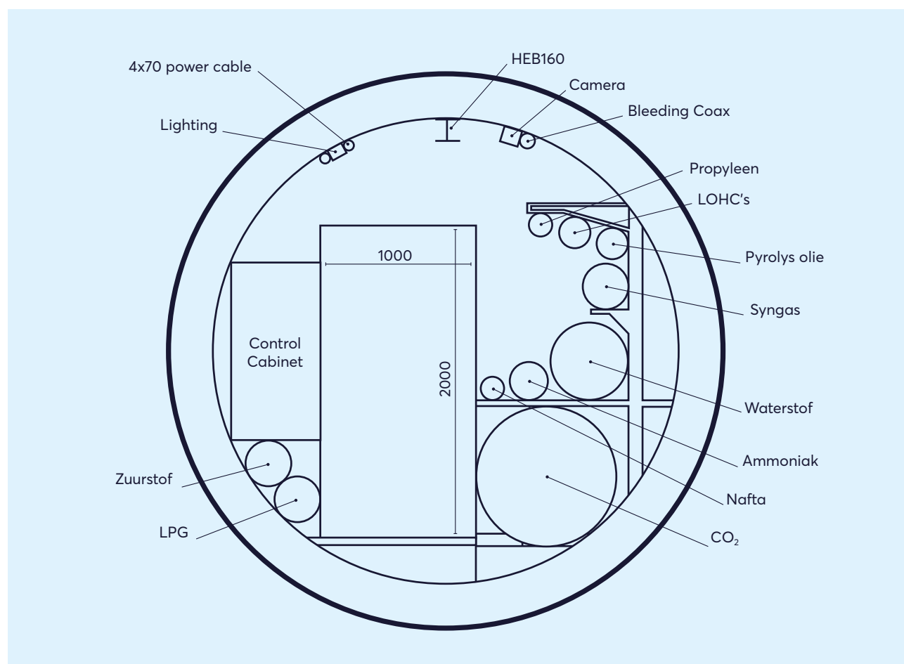
Figuur 5: Tekenskets dwarsdoorsnede van een 3-meter MUK (Arcadis, 2025)
