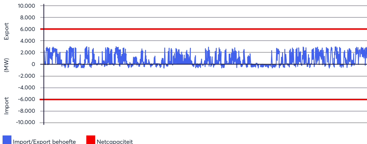
Figuur 29: Knelpuntenanalyse uurniveau exportcapaciteit (2a + SF, basisjaar 2040)
