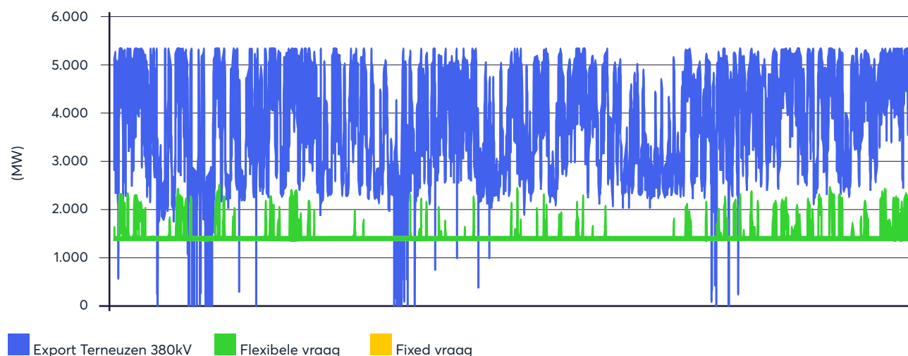
Figuur 48: Locatiesturing vraagstimulering Terneuzen – Rilland
