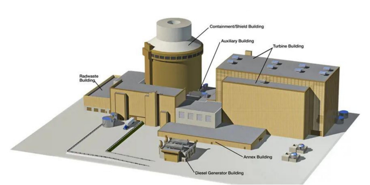
Figuur 3-2: indicatieve visualisatie van één EPR reactor (bron: EDF energy).
